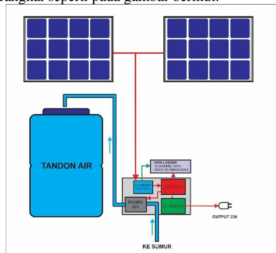
Gambar 6. Rangkaian Pompa Air Tenaga Surya
