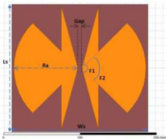
Gambar 1. Rancangan Antena
